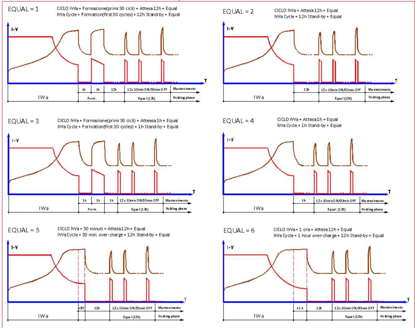
Fig.4: Caratteristiche dei cicli di carica con egualizzazione
