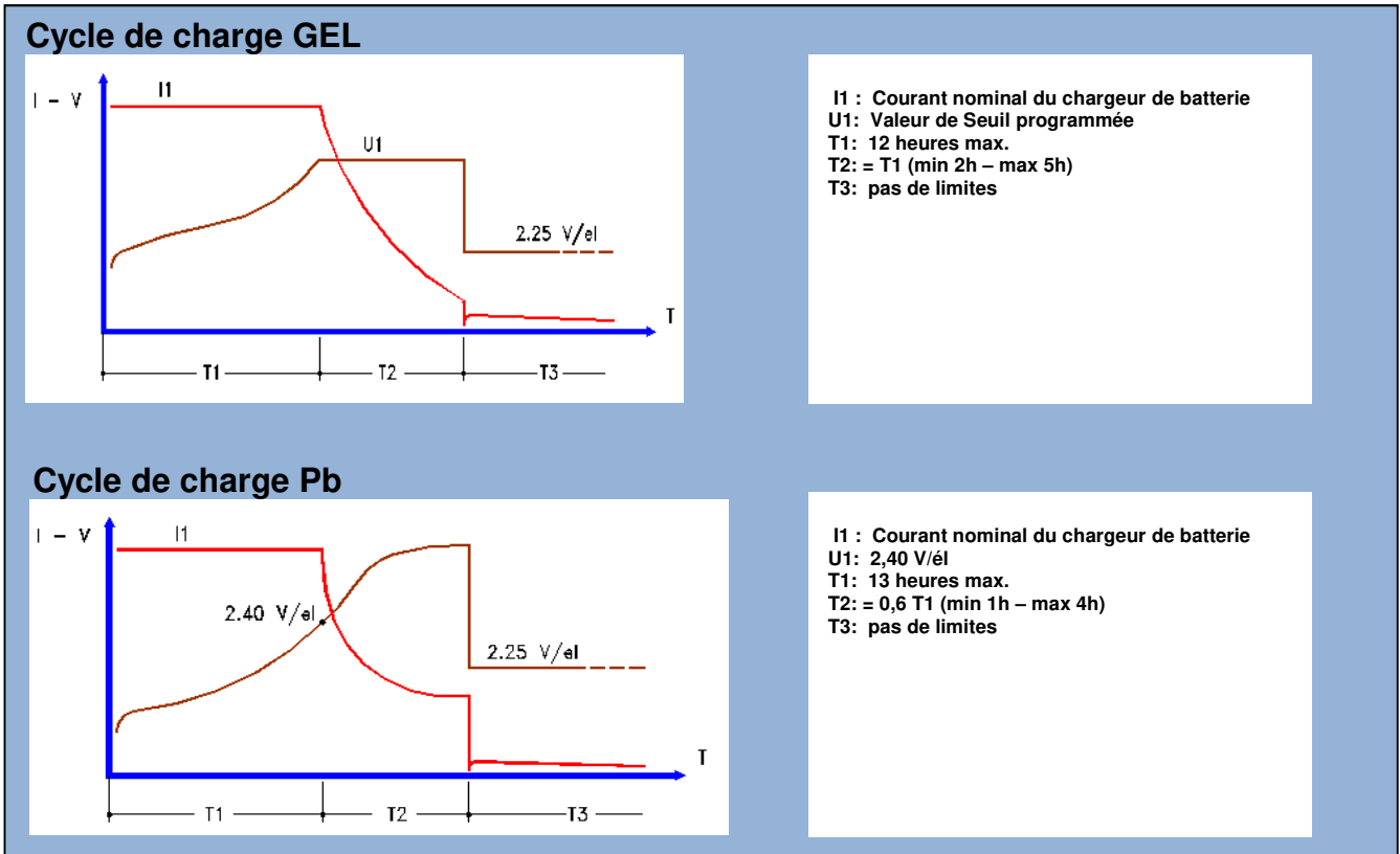
Fig.2: Graphiques des courbes de charge disponibles sur les chargeurs de batterie MGX
