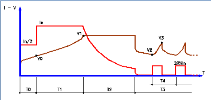
Fig.1: Graphiques des courbes de charge disponibles sur les chargeurs de batterie PSW et ZHF
